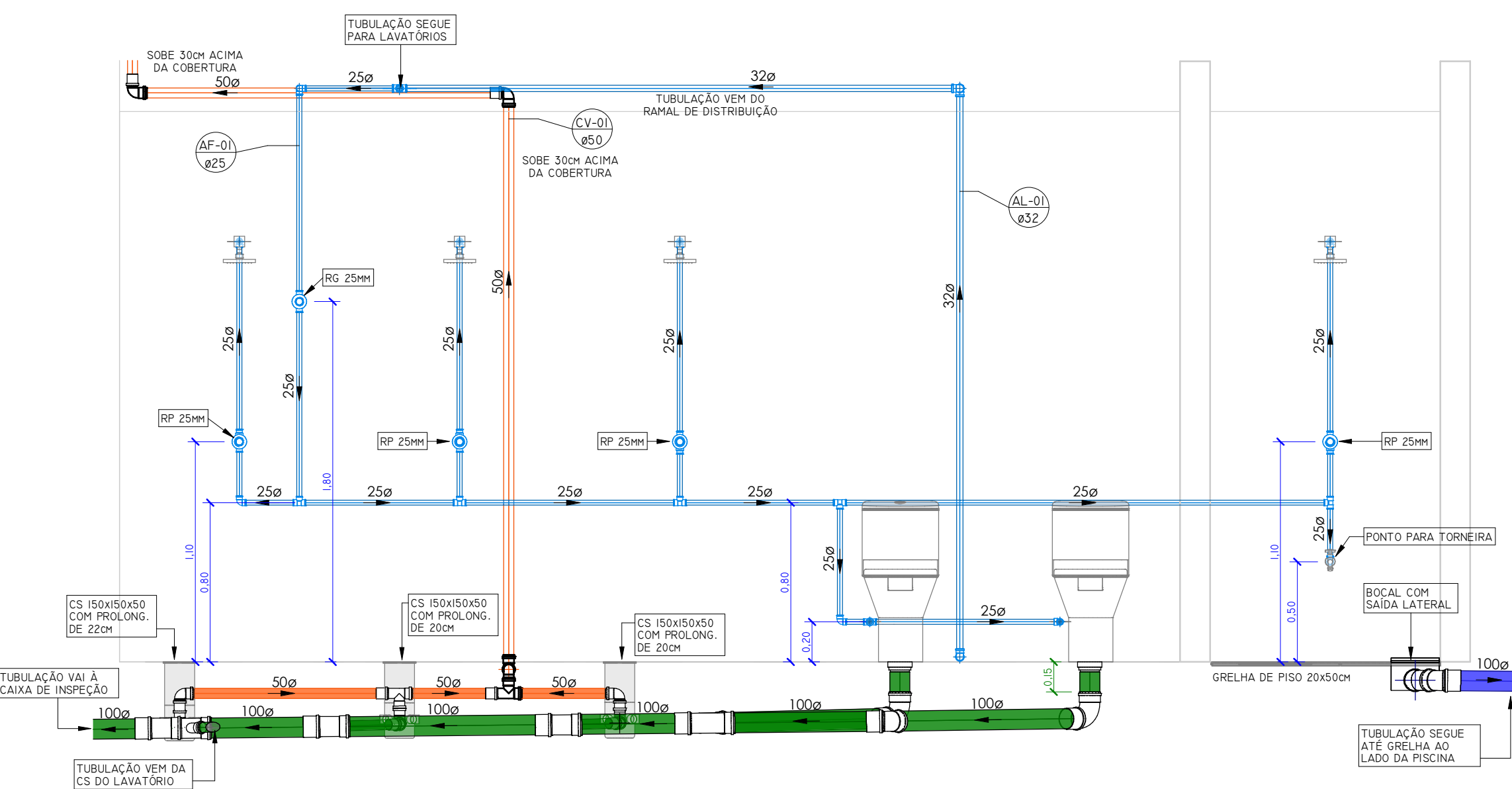
VISTA FRONTAL SANITÁRIO FEMININO E DUCHA ESCALA 1 : 25
