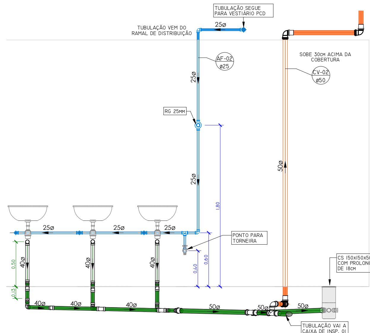
VISTA FRONTAL LAVATÓRIO FEMININO ESCALA 1 : 25
