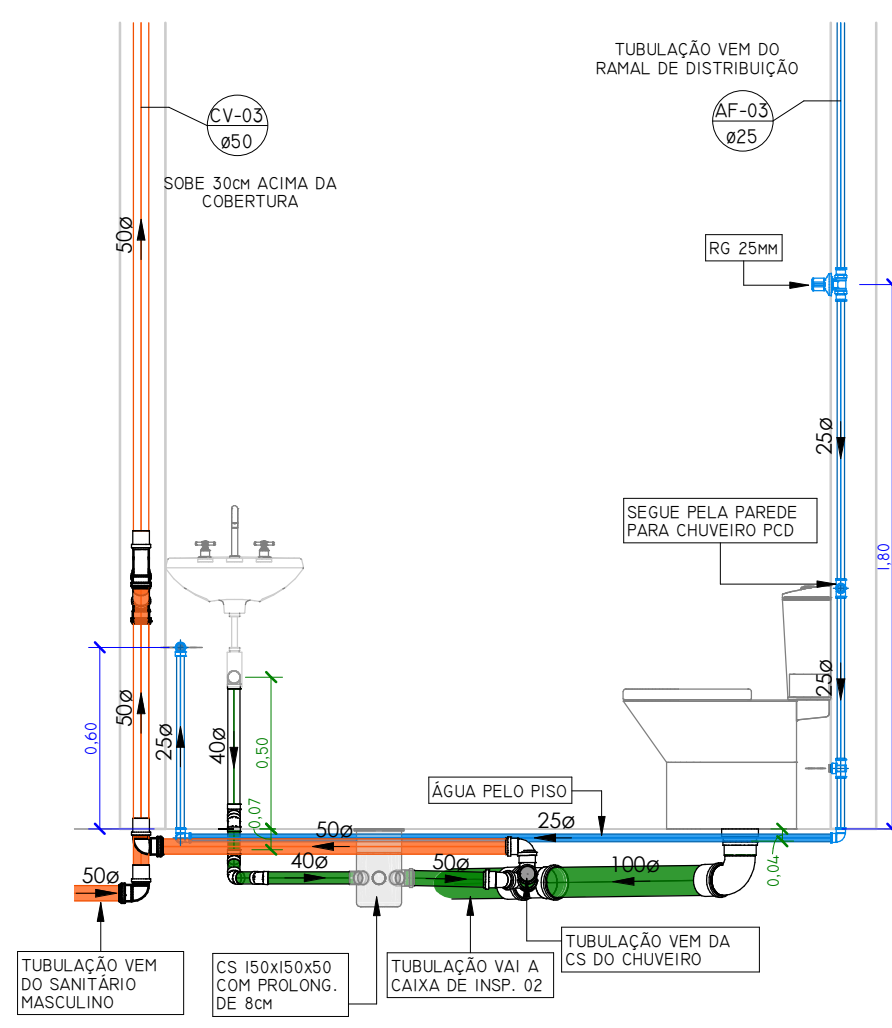
VISTA FRONTAL BS E LAVATÓRIO PCD ESCALA 1 : 25
