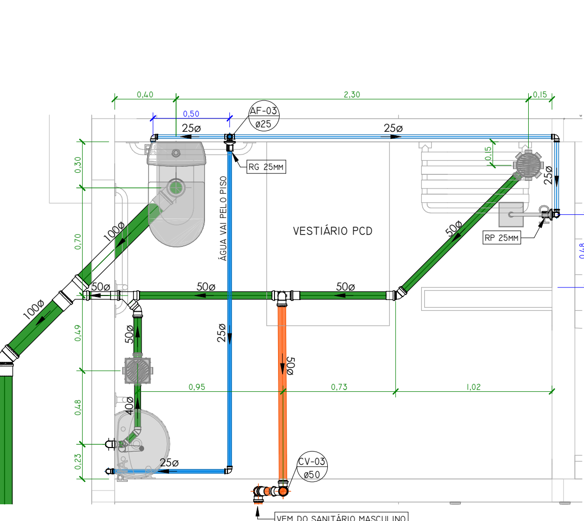
PLANTA BAIXA VESTIÁRIO PCD ESCALA 1 : 25
