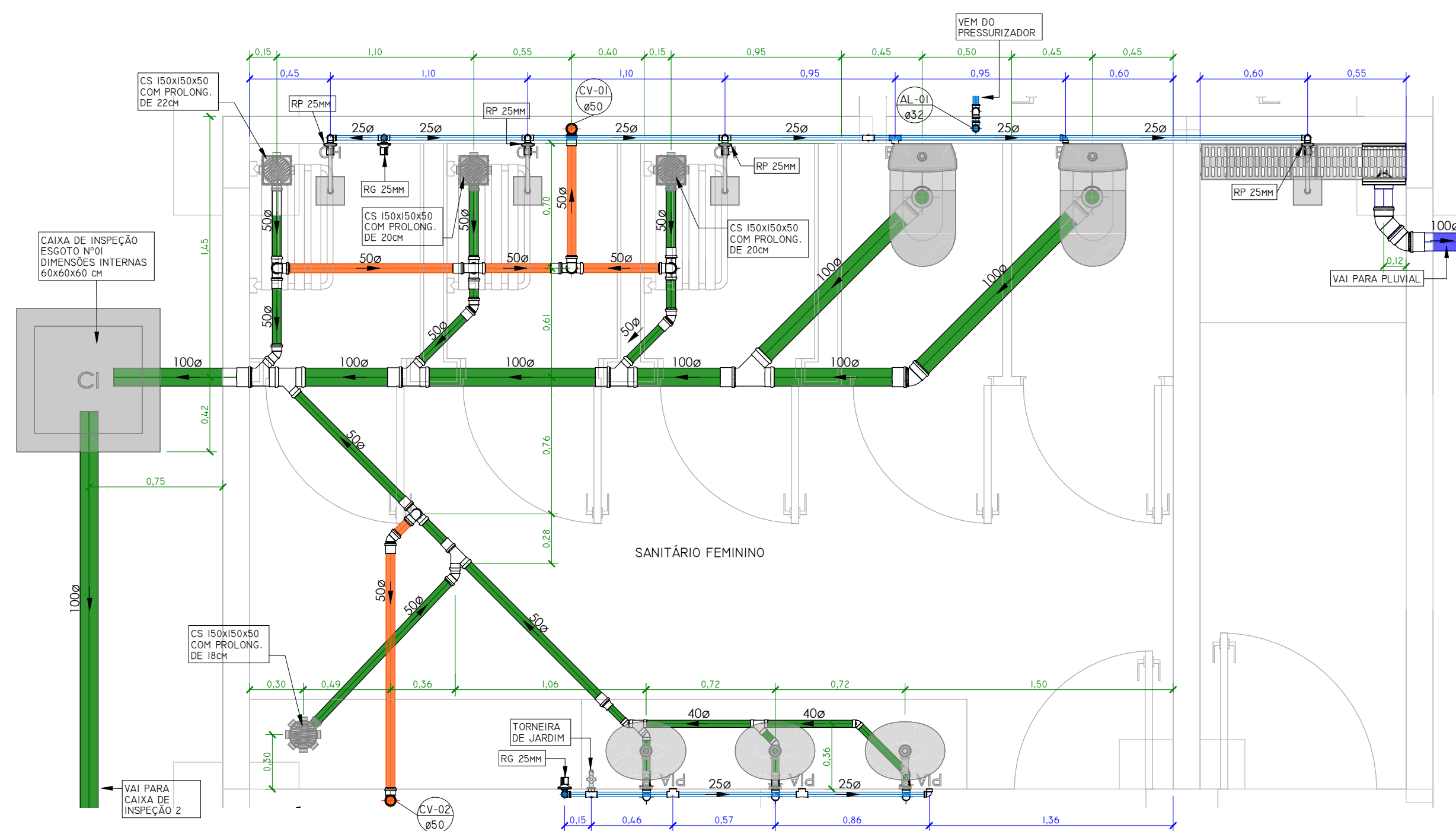
PLANTA BAIXA SANITÁRIO FEMININO E DUCHA ESCALA 1 : 25
