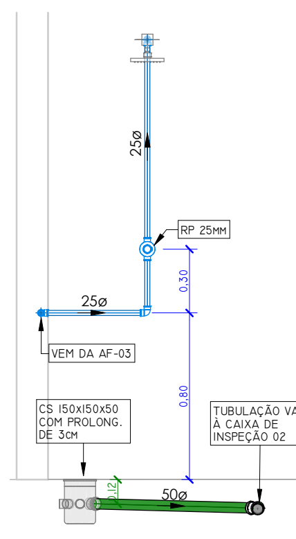
VISTA FRONTAL CHUVEIRO PCD ESCALA 1 : 25
