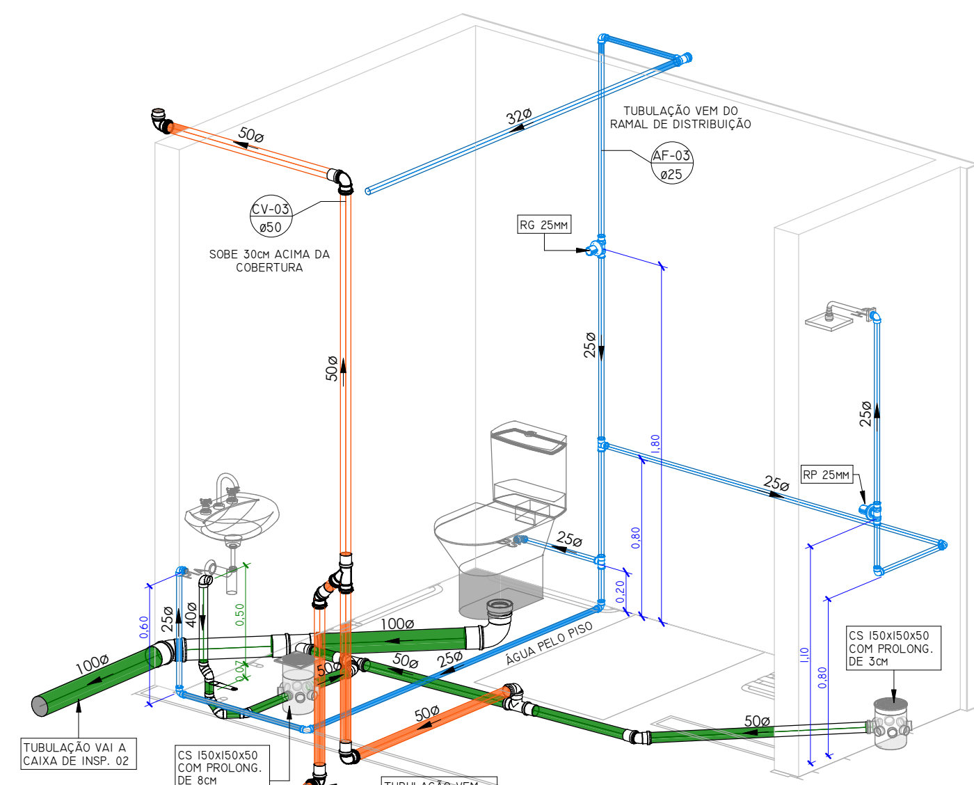
DETALHAMENTO VESTIÁRIO PCD
