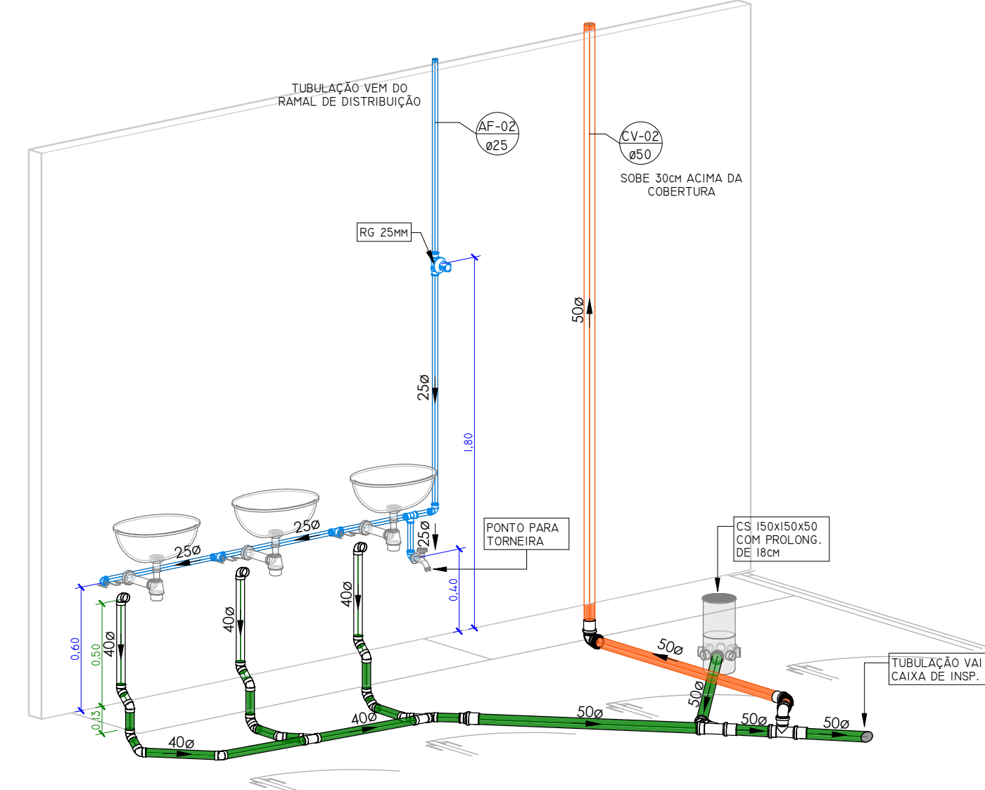
DETALHAMENTO LAVATÓRIO FEMININO
