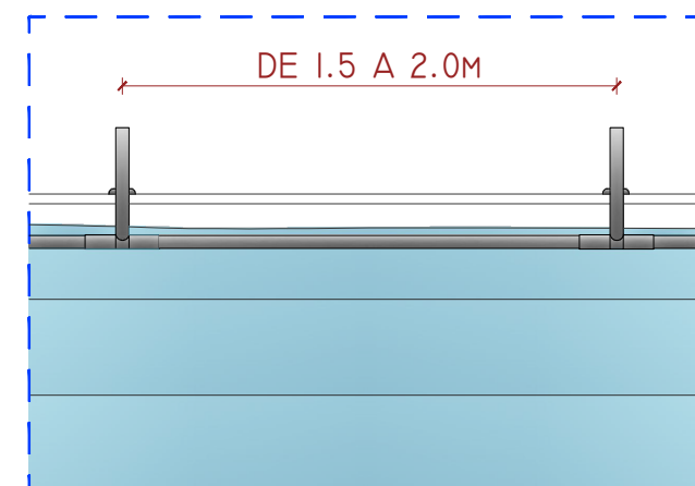
DET. 03 - VISTA FRONTAL CORRIMÃO PISCINA ESCALA: 1/25
