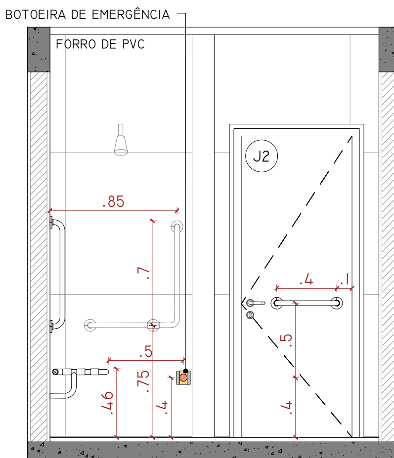
DET. 01 - V03 SANITÁRIO PCD ESCALA: 1/25
