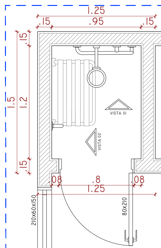
DET. 01 - PB. SANITÁRIO PCD ESCALA: 1/25
