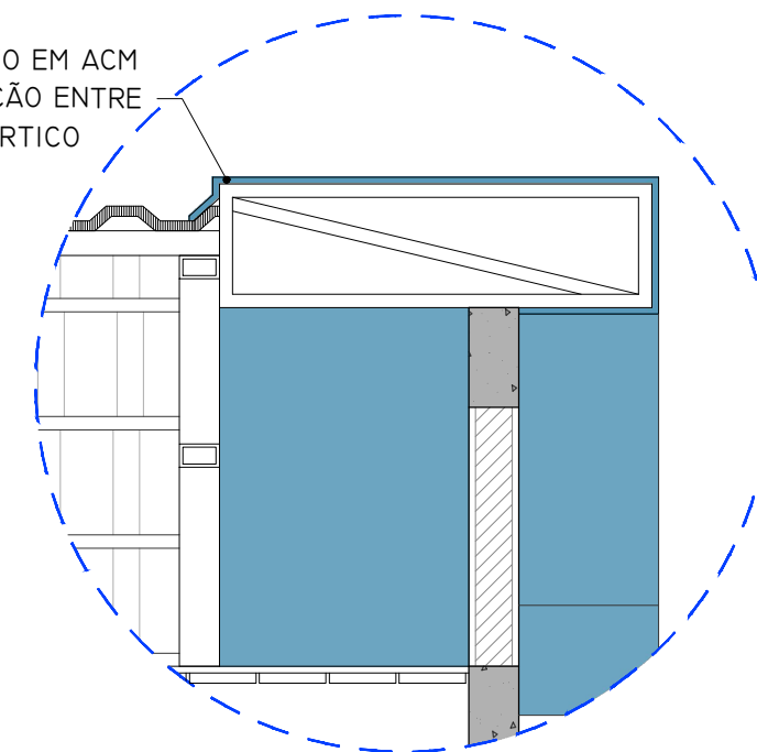
DET. 06 - PÓRTICO ACM ESCALA: 1/25
