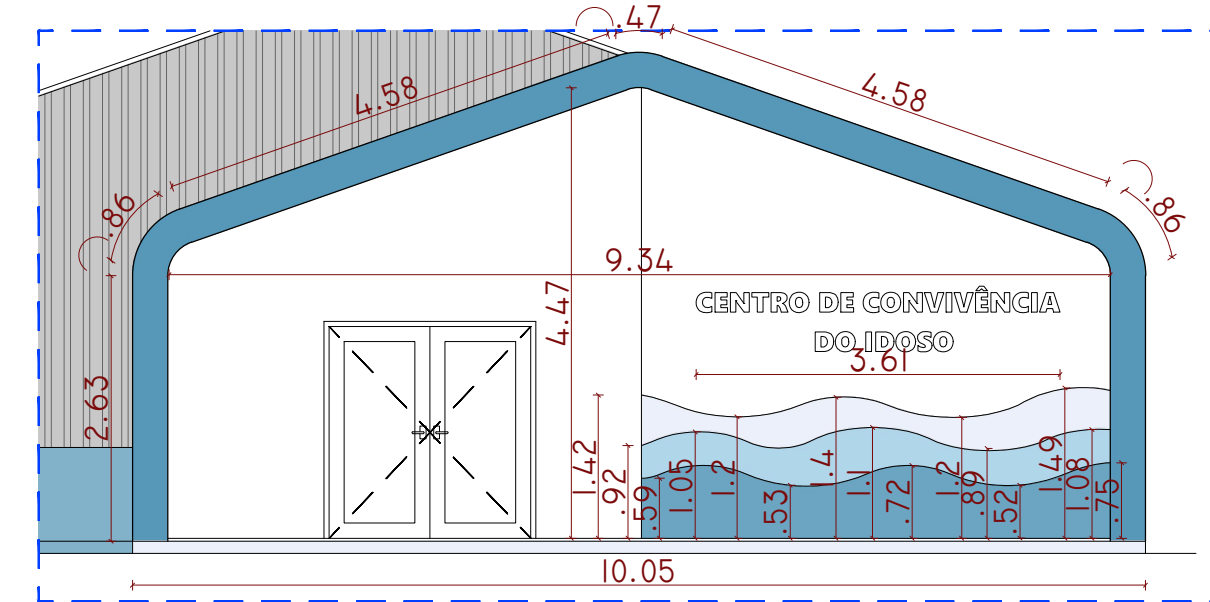
DET. 08 - PÓRTICO E ONDAS EM ACM ESCALA: 1/75
