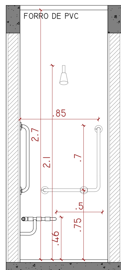
DET. 02 - V01 CHUVEIROS ESCALA: 1/25
