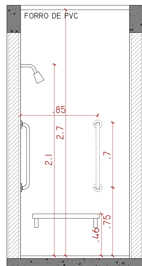
DET. 02 - V02 CHUVEIROS ESCALA: 1/25
