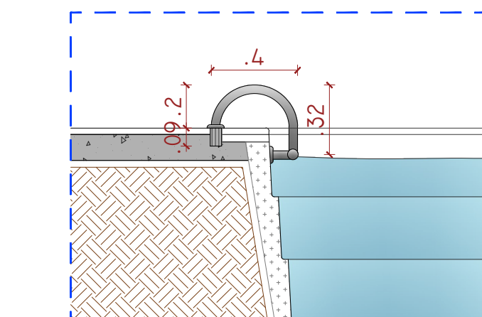
DET. 03 - VISTA LATERAL CORRIMÃO PISCINA ESCALA: 1/25
