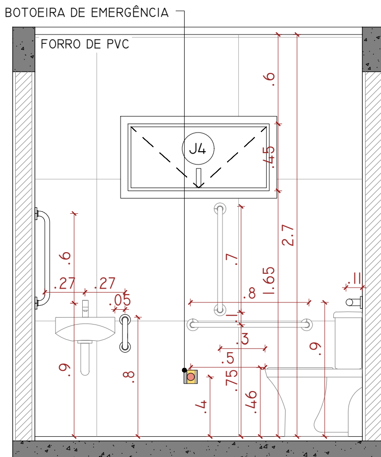
DET. 01 - V01 SANITÁRIO PCD ESCALA: 1/25
