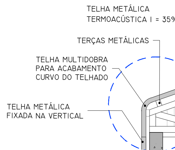
DET. 07 - ACABAMENTO COBERTURA ESCALA: 1/25
