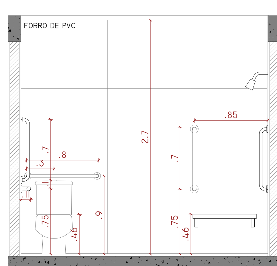
DET. 01 - V02 SANITÁRIO PCD ESCALA: 1/25
