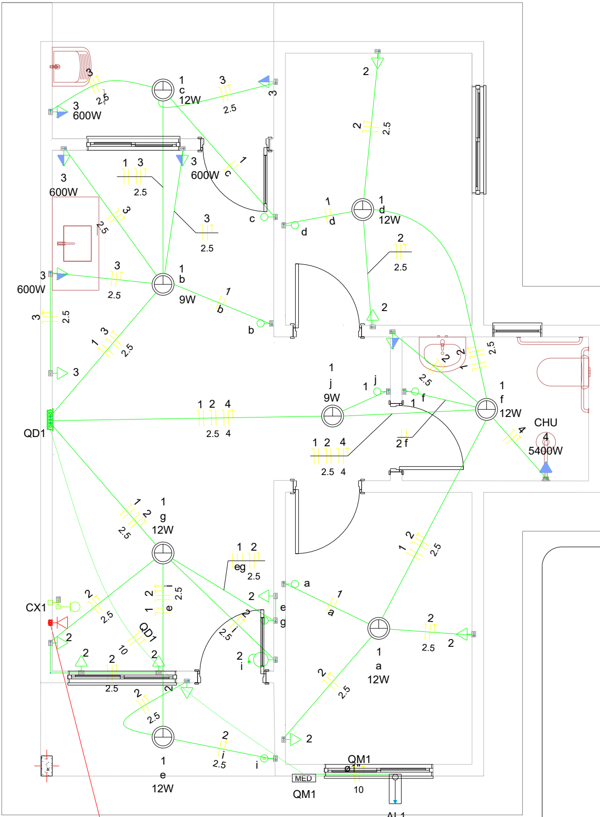
PROJETO ELÉTRICO - PLANTA BAIXA ESCALA 1:100
