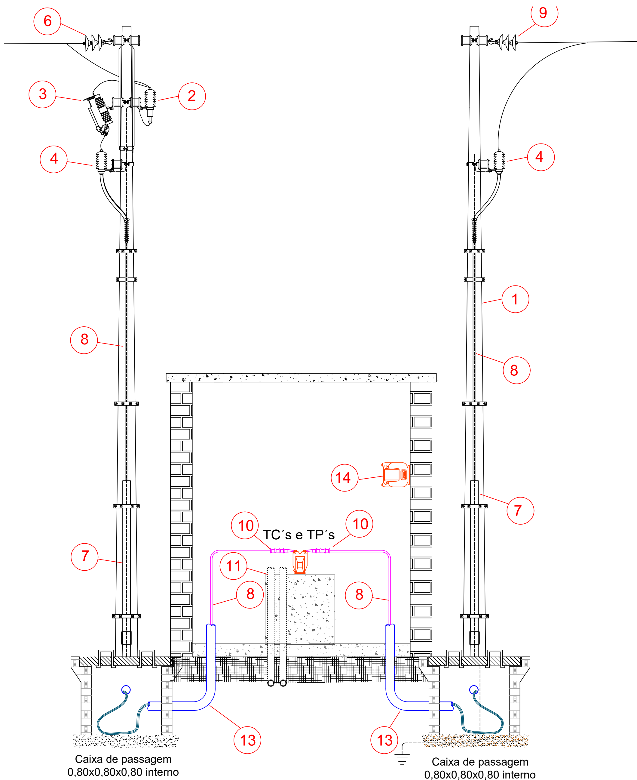
CORTE AA ESC.1/25
